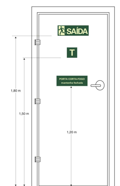
Figura 3 - Sinalização de porta corta-fogo do térreo (vista da escada)
