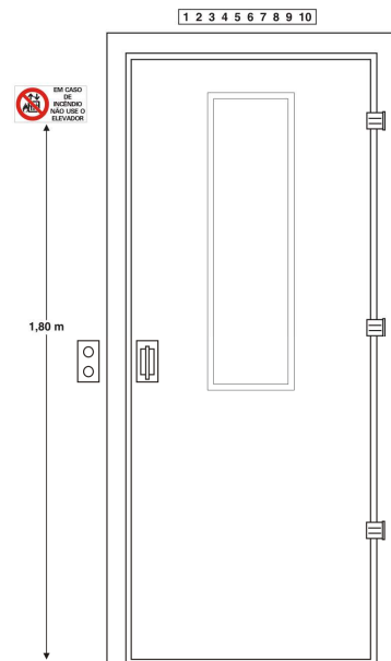
Figura 4 - Sinalização de elevadores
