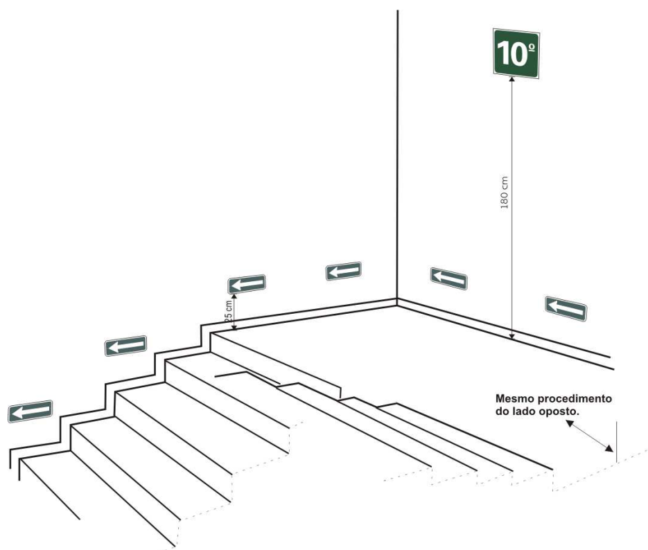
Figura 8 - Sinalização complementar. Exemplo de rodapé.
