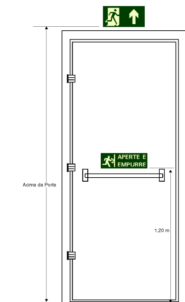
Figura 5 - Sinalização de portas com barras antipânico (modelos 1 e 2)
