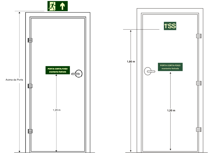
Figura 1 - Sinalização de porta corta-fogo (vista da escada) Figura 2 - Sinalização de porta corta-fogo (vista do hall)
