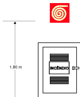
Figura 7 - Sinalização de hidrante
